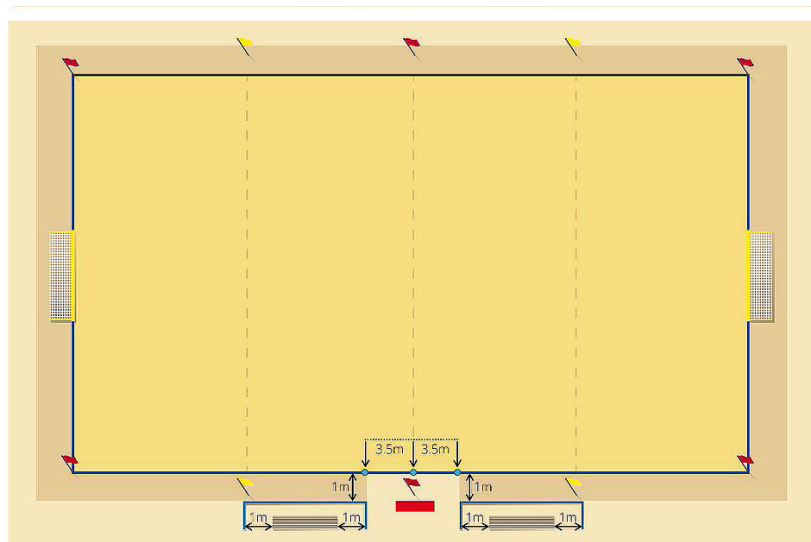
Рисунок 69. Зона замены.
