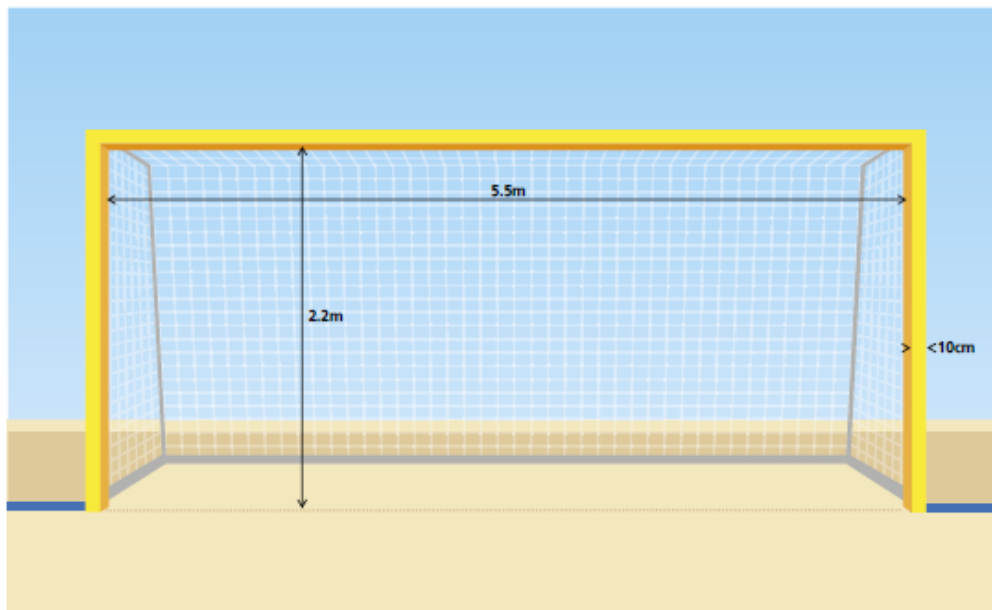
Рисунок 71. Размеры ворот.
