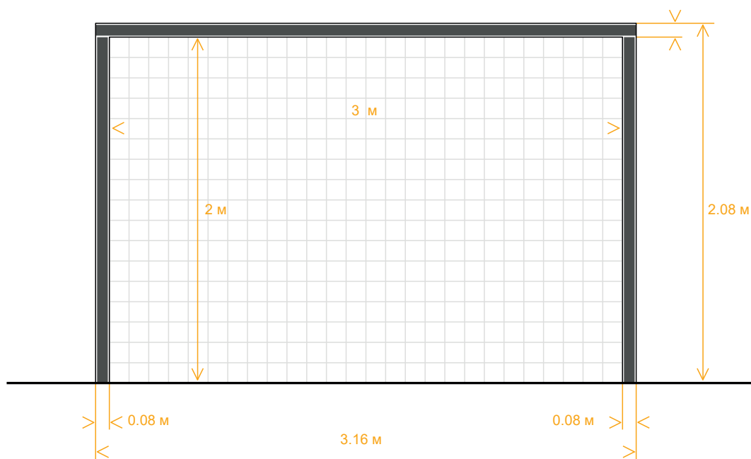
Рисунок 19. Размеры ворот.
