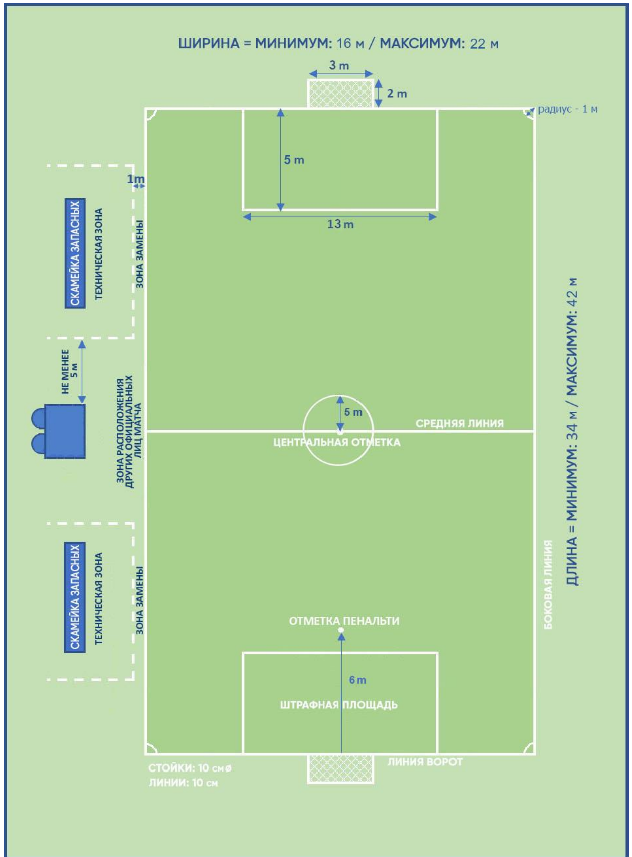
Рисунок 107. Маркировка, размеры и оборудование поля.
