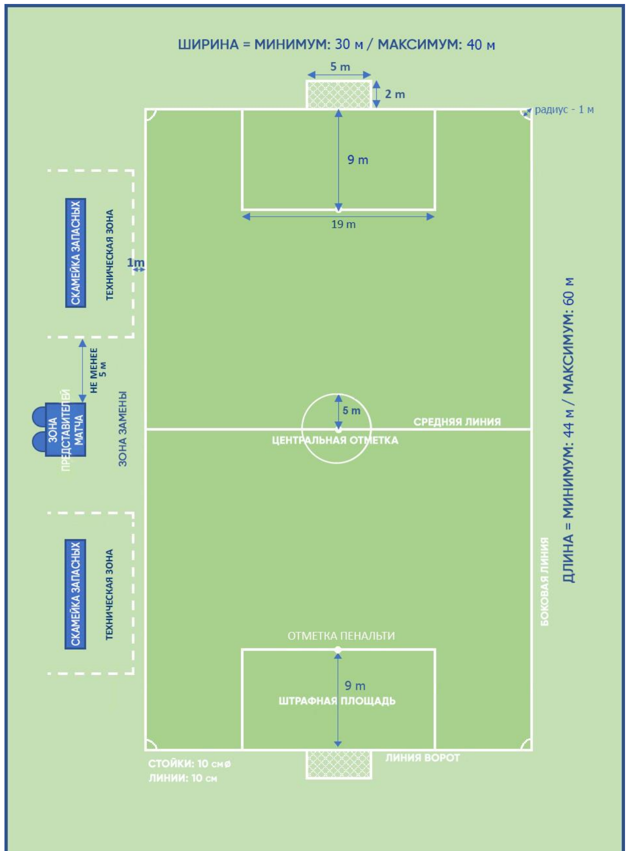
Рисунок 101. Маркировка, размеры и экипировка игрового поля.
